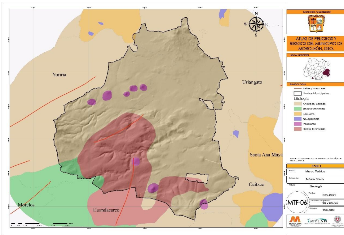
Mapa 5 Litología de Moroleón
